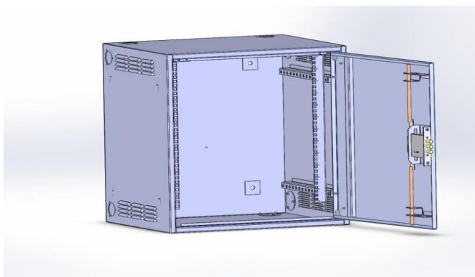
Рис.1 Примерный вид шкафа (размеры указаны в таблице №1)
