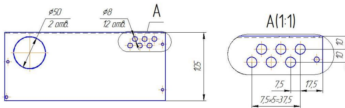
Рисунок 2. Задняя стенка КБ/КЯ (ЯР) с расположением крепежных ( d=8 мм) и монтажных ( d=4 мм) отверстий под опору/раму с плитами.
