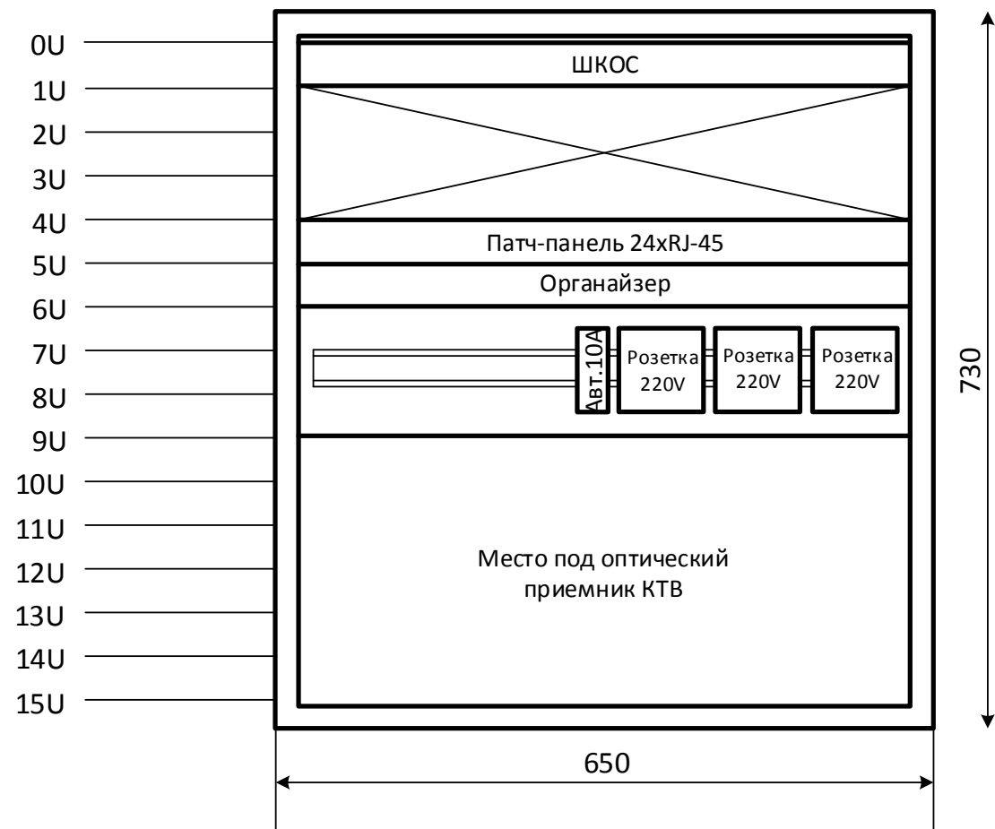
Рис.2 Чертеж шкафа.
